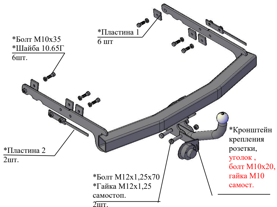
Рис.1 Тягово-сцепное устройство 6020
